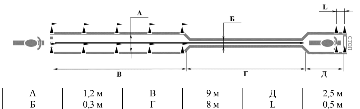
Рисунок 2. Схема и размеры упражнения № 2
